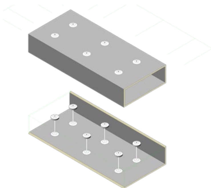
Applicazione con 2 barre di rinforzo ogni 600 mm
