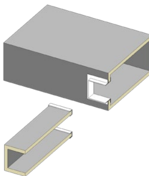
Connessione con profili
