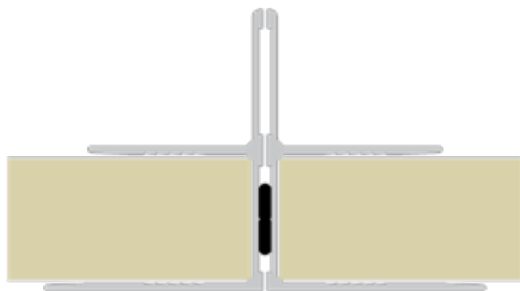
Sistema di connessione a profili in alluminio.
