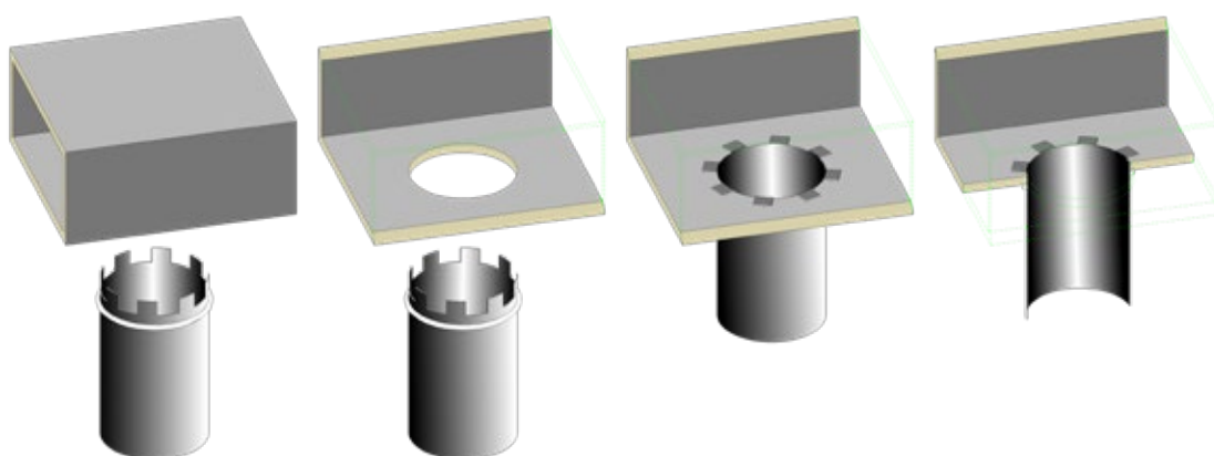
Installazione di un collarino a spirale
