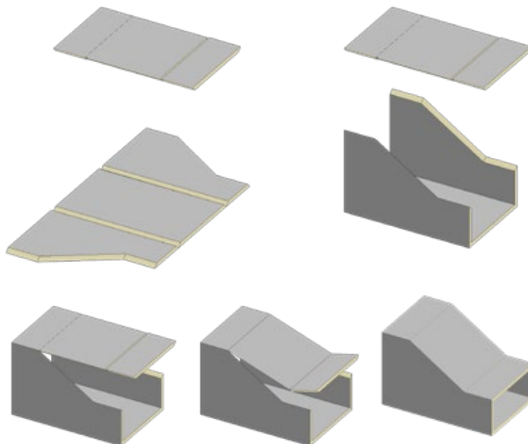
Deviazione a Stivale
